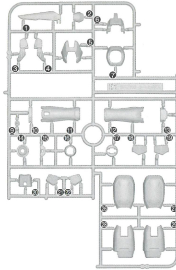
B1パーツ (スチロール樹脂: PS)
